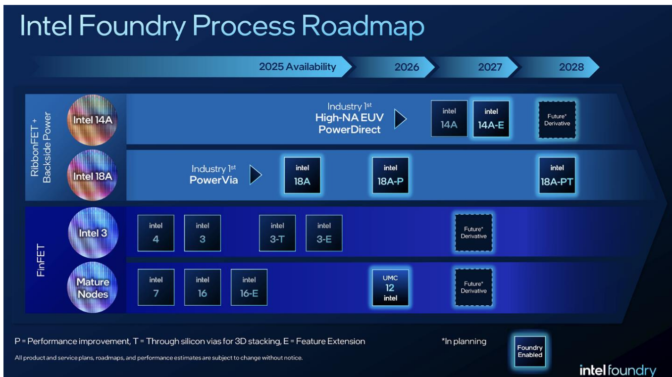
图表2：英特尔制程路线图
